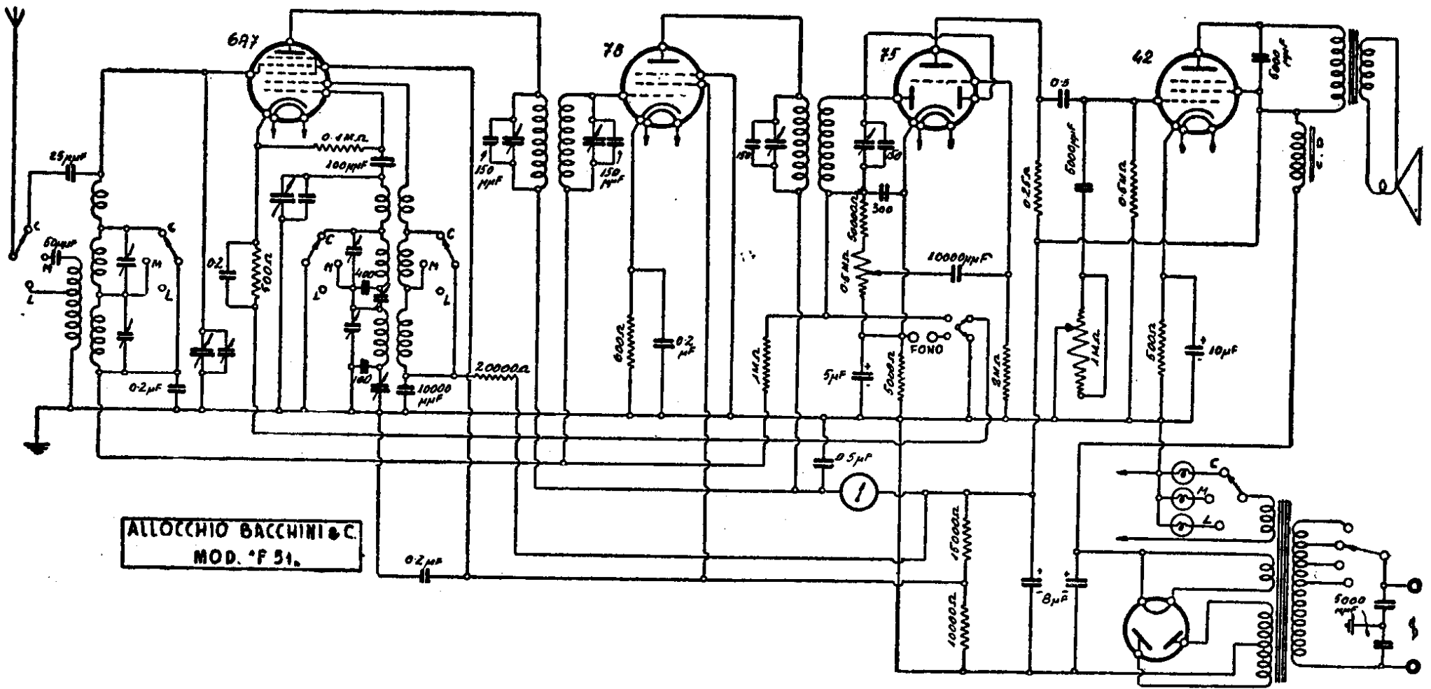
ALLOCCIO. BACCHINI e Co. — Mod. 51 F.M. e Mod 51 G Produzione 1936. - Media freq.: 425 kc.
